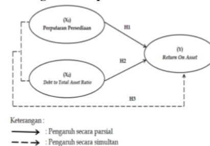
Gambar1. Kerangka Konseptual
